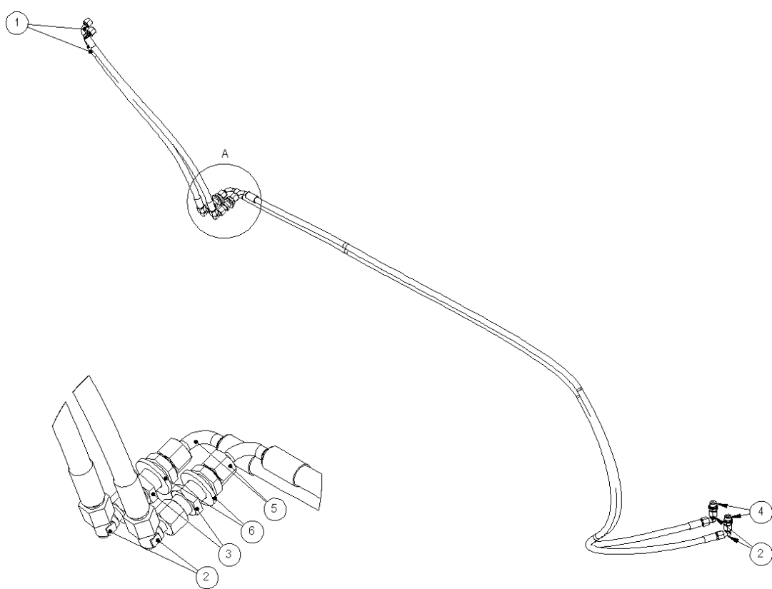
DETAIL A 1 : 2
