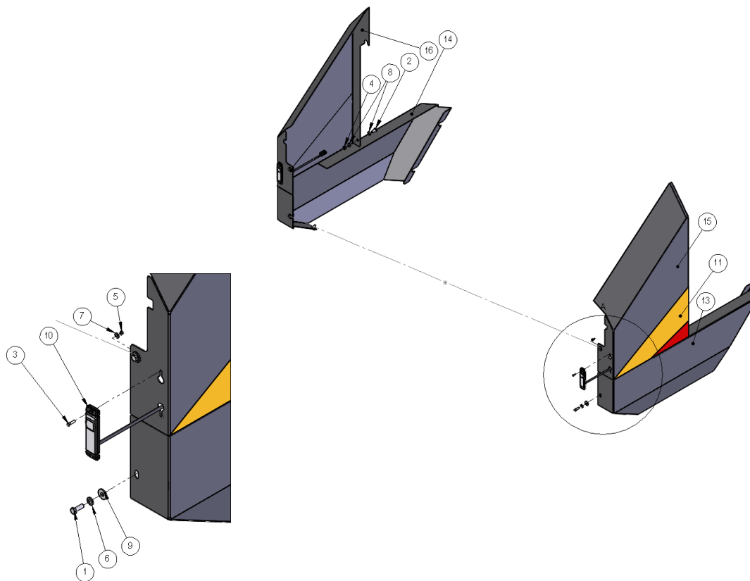
DETAIL A 1 : 5
